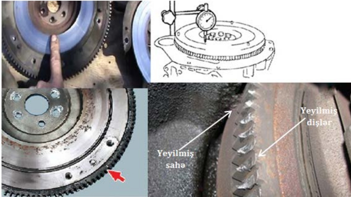
Şəkil 1.9. Nazım çarxın yoxlanılması
