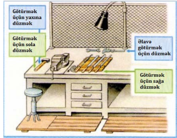
Şəkil 6.2. İşçi yerində alətlərin saxlanması və rahat istifadəsi üçün avadanlıq. İşçinin ayaq altına taxta ayaqaltı qoyulur
