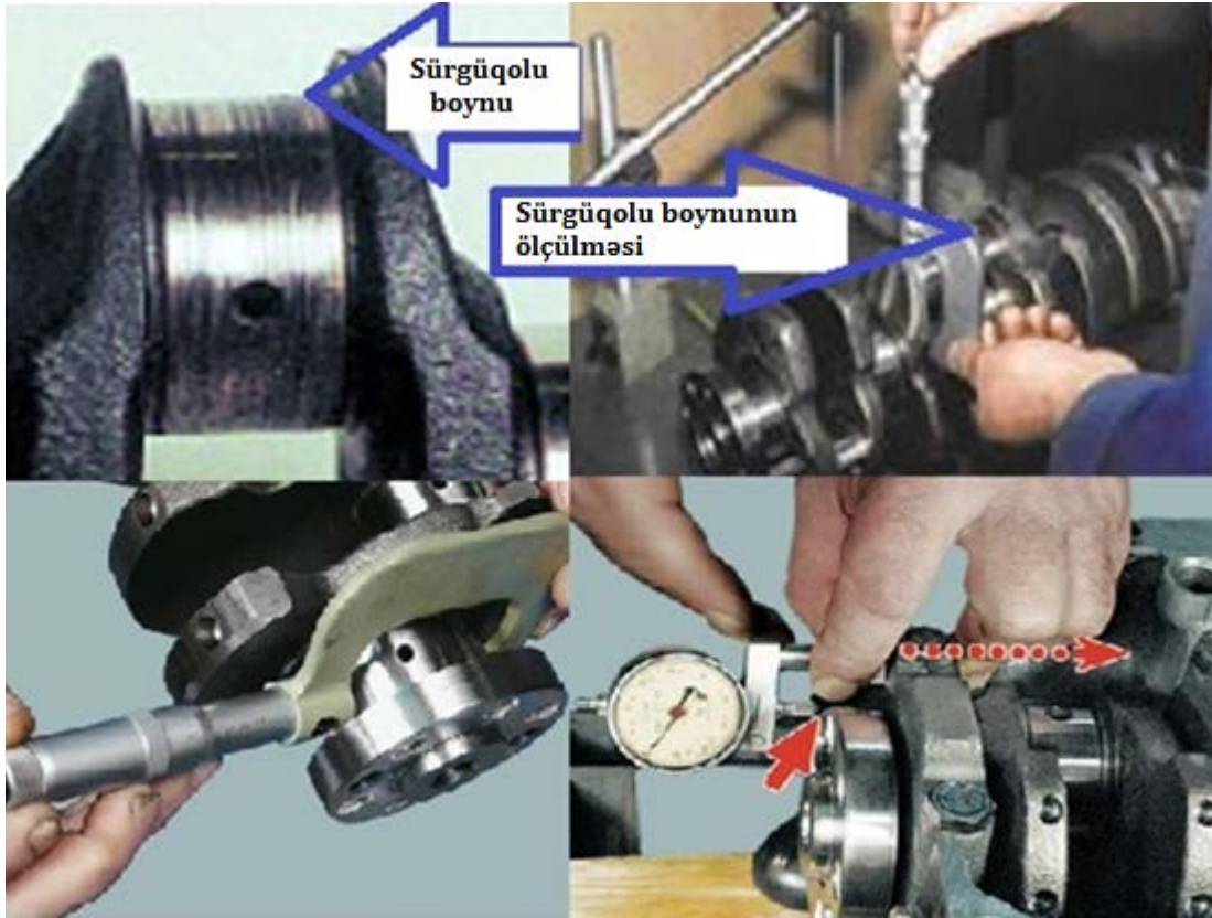
Şəkil 1.8. Dirsəkli valın yoxlanması
