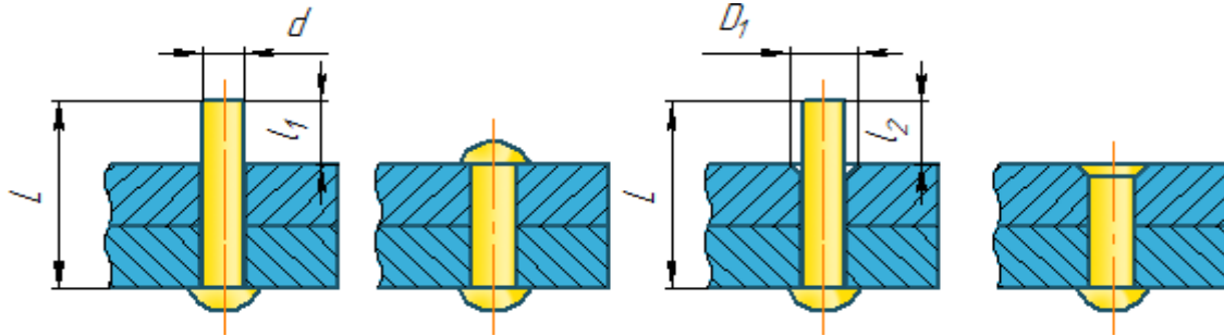
Şəkil 5.26. Birləşmənin təyin olunmuş uzunluğu
