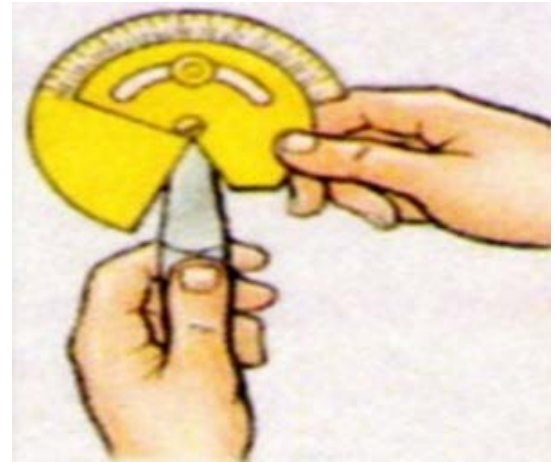
Şəkil 4.12. İskənənin itilik bucağının yoxlanması
