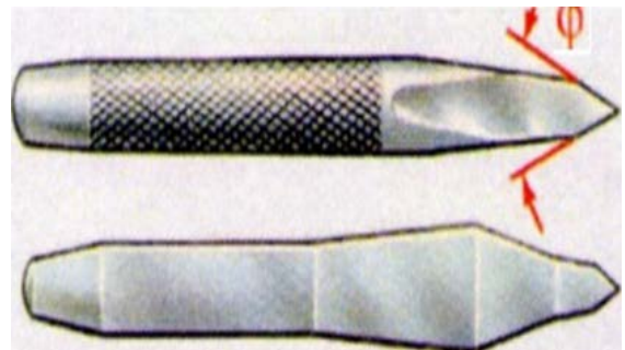
Şəkil 4.10. İskənənin itilik bucağının göstərilməsi
