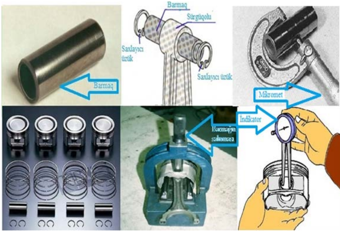
Şəkil 1.2. Porşen barmaqının yoxlanılması
