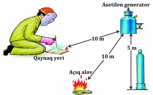
Şəkil 6.39. Qaynaq zamanı təhlükəsiz ara məsafəsinin təmin olunması
