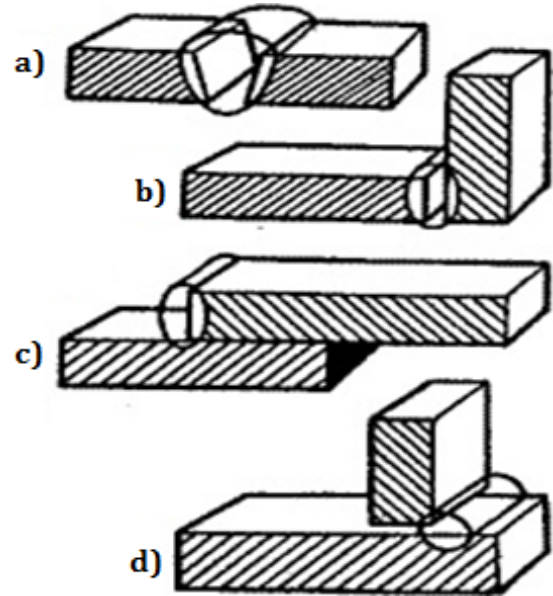
Şəkil 2.56. Metal hissələrin qaynaqla birləşdirilməsi
