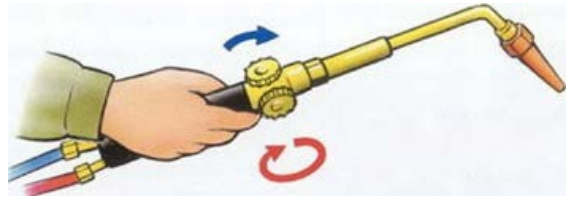
Şəkil 3.19. Yandırılacaq qaz qarışığı təzyiqinin nizamlanması
