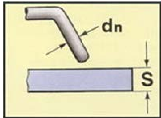
Şəkil 3.23. Doldurucu naqilin diametrinin seçilməsi
