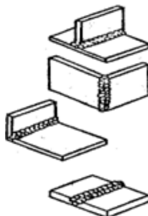
Şəkil 2.61. Bərk lehimləmə ilə hissələrin birləşdirilməsi
