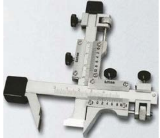
Şəkil 1.31. Dişölçənlər
