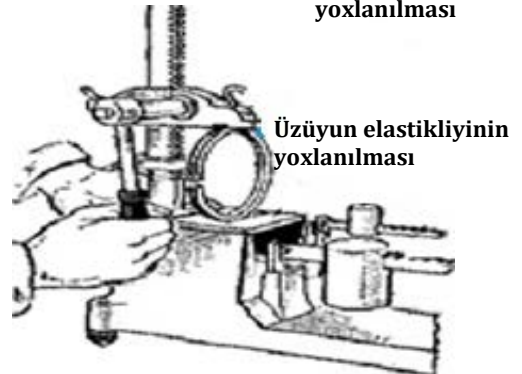
Şəkil 1.3. Porşen üzüyünün yoxlanılması
