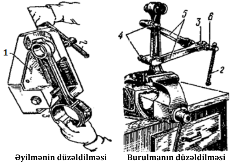
Şəkil 1.3. Sürgüqolunun düzləndirilməsi
