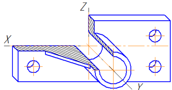
Şəkil 5.4. Hissədən bir hissənin kəsilib çıxarılması
