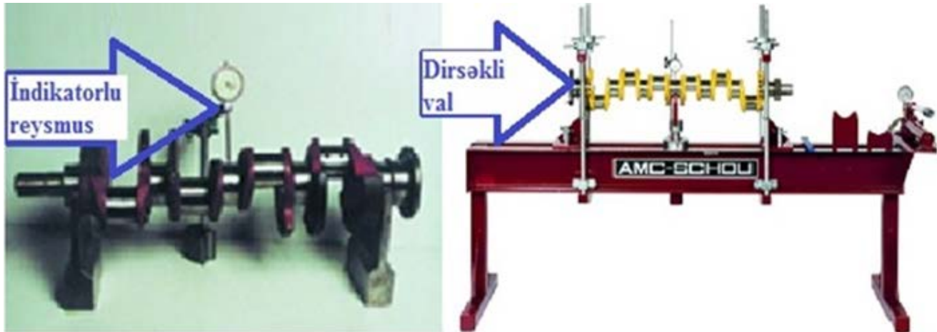
Şəkil 1.7. Dirsəkli valın əyriliyinin yoxlanması.
