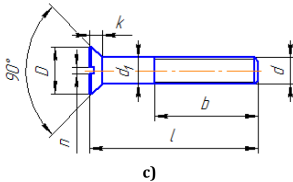
Şəkil 5.24. Yivli birləşmələrdə istifadə olunan şurupların sxematik təsviri
