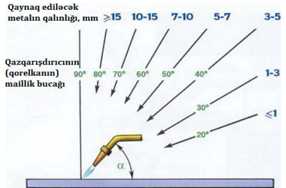
Şəkil 3.26. Qaynaq ediləcək metalın qalınlığından asılı olaraq qalyanın maillik bucağının seçilməsi
