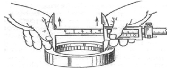
Şəkil 1.28. Ştangenpərgarla hissənin daxildən ölçülməsi
