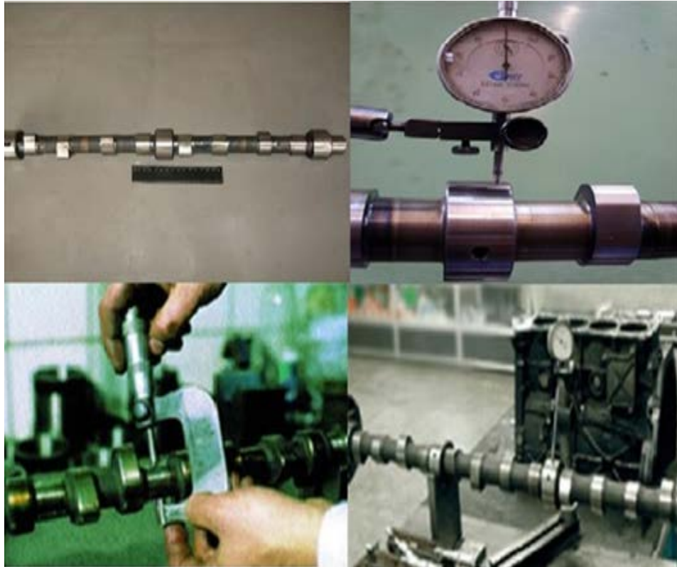
Şəkil 1.11. Yumuruqlu valın yoxlanması
