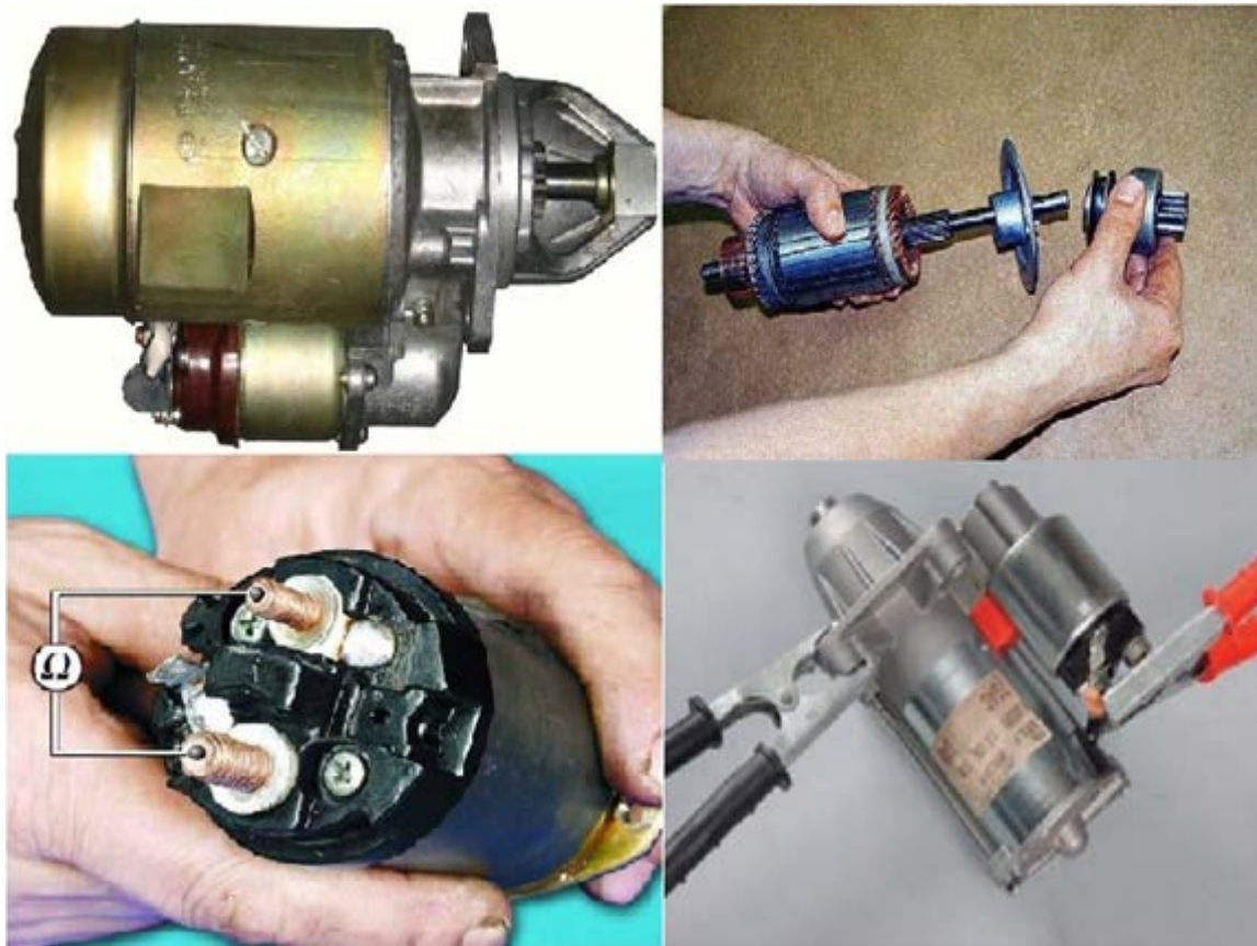
Şəkil 1.20. Starterlərin yoxlanılması
