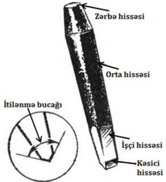
Şəkil 4.9. İskənə
