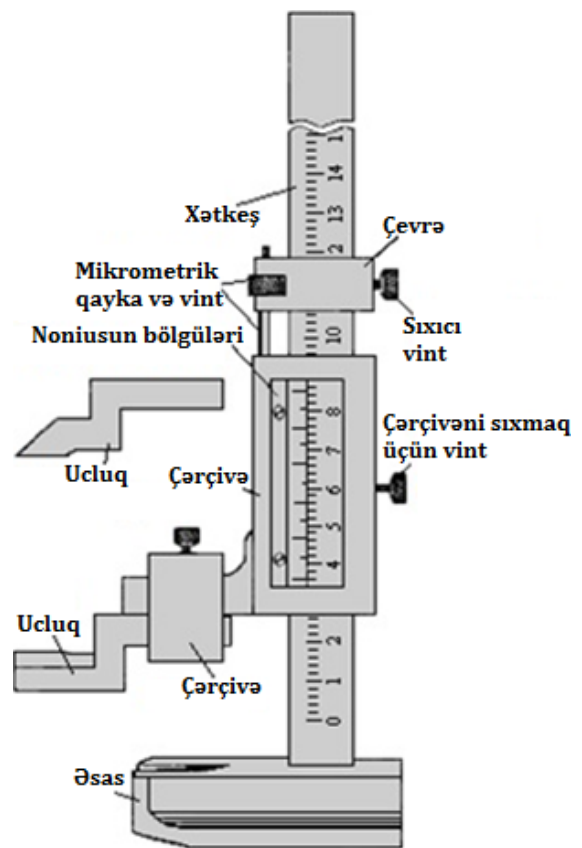
Şəkil 1.34. Ştangenreysmus
