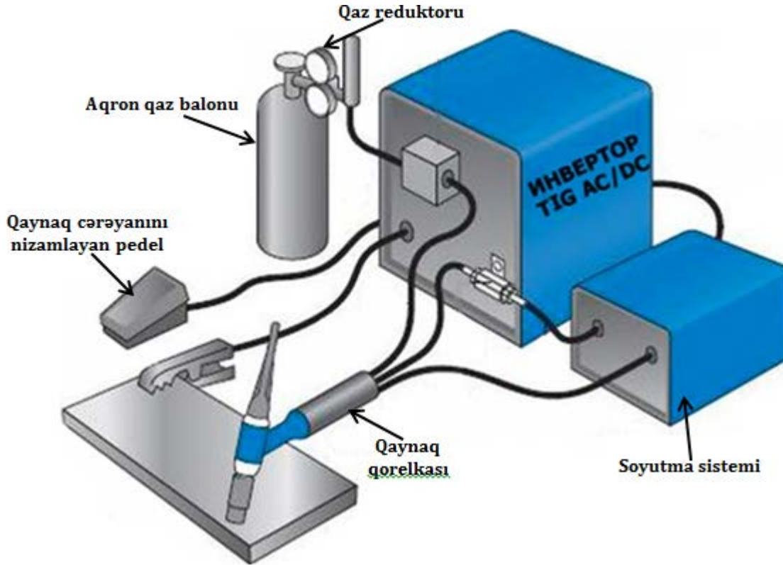
Şəkil 3.8. Arqon qaz daxilində alüminium hissələrin qaynaq edilməsi üçün aparat
