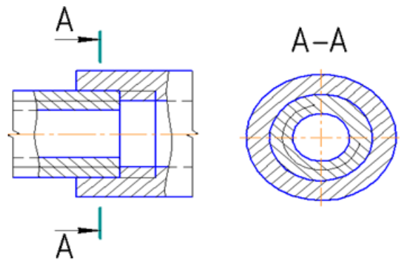
Şəkil 5.23. Deşikdə görülməyən yivin kəsimdə çəkilmiş formada təsviri
