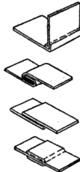
Şəkil 2.60. Yumşaq lehimləmə ilə hissələrin birləşdirilməsi
