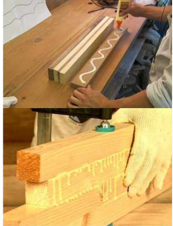
Şəkil 2.63. Ağacın yapışqanla birləşdirilməsi
