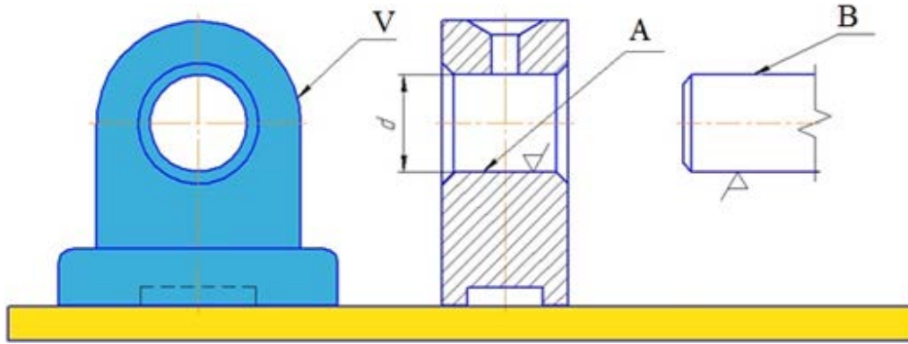
Şəkil 5.13. Sərbəst ölçülər.
