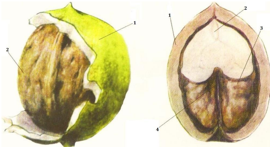
Şəkil 1.12. Cəvizin ( Juglans regia ) meyvəsinin quruluşu
