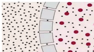
Şəkil 1.3. Osmos prosesinin mexanizmi
