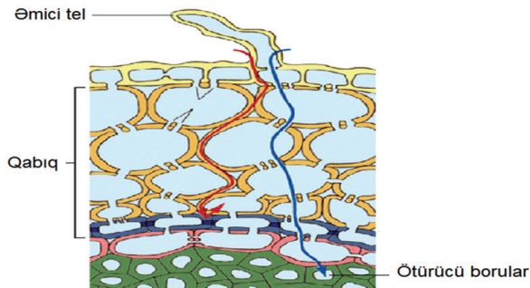
Şəkil 2.1. Bitkilərin kök vasitəsilə qidalanması
