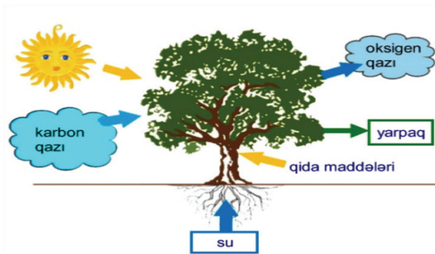
Şəkil 2.2. Bitkilərin qidalanması mexanizmi
