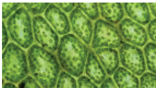
Şəkil 1.5. Xlorofilin mikroskopla görüntüsü
