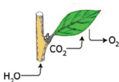
Şəkil 1.6. Fotosintez prosesinin reaksiyası
