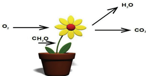
Şəkil 1.7. Bitkilərin tənəffüs sxemi
